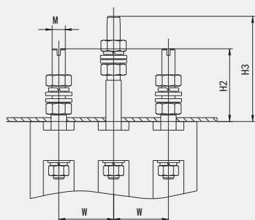
三极 HYM3L-125、160 板后接线外形及安装尺寸
