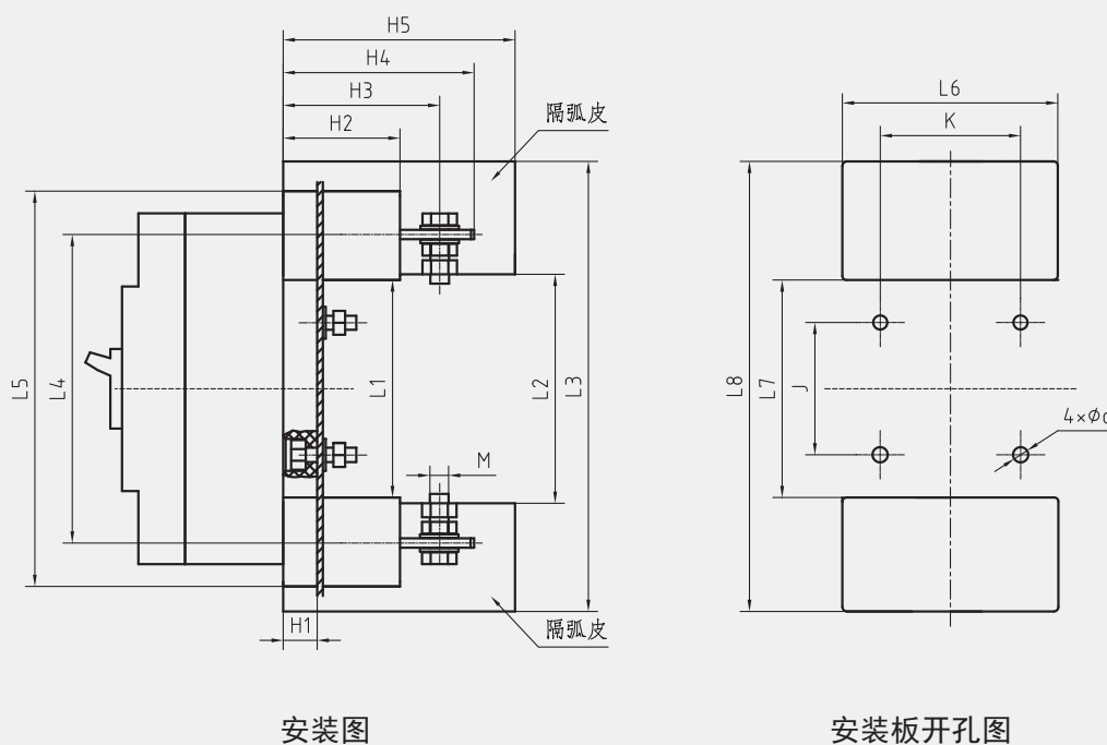
3P插入式安装尺寸
