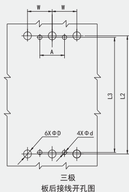
三极 板后接线开孔图
