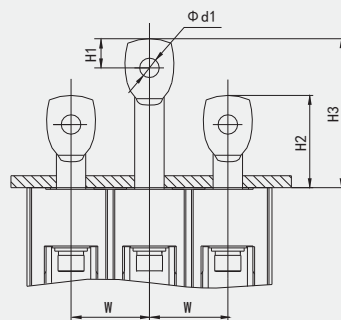
三极 HYM3L-250、400、630、800板后接线外形及安尺寸
