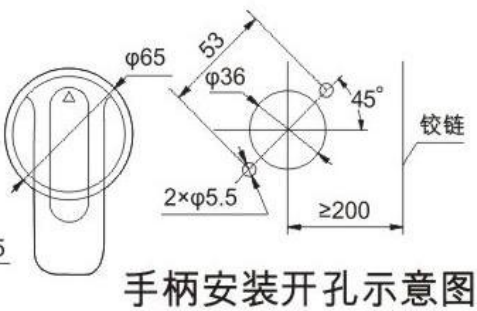
图 5 手动操作机构安装尺寸
