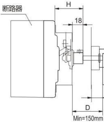
图 4 电动操作机构安装尺寸
