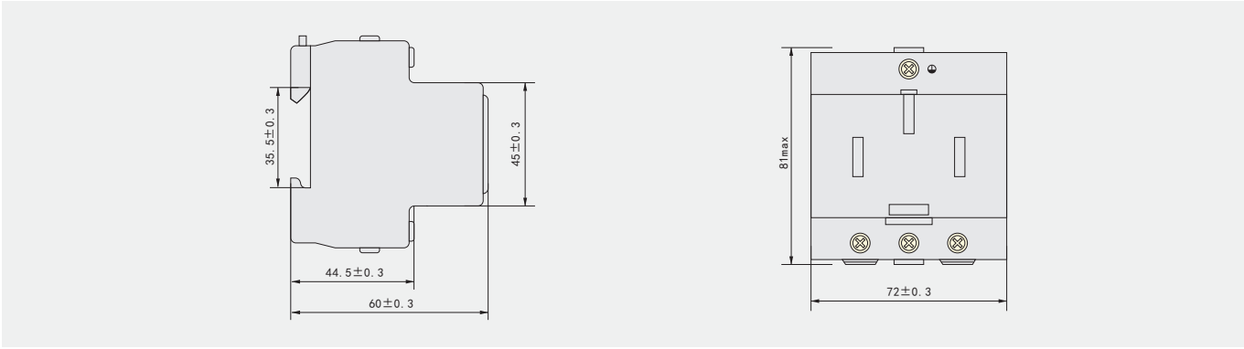
图 5、AC30-10 (16) /5 250~外形及安装尺寸
