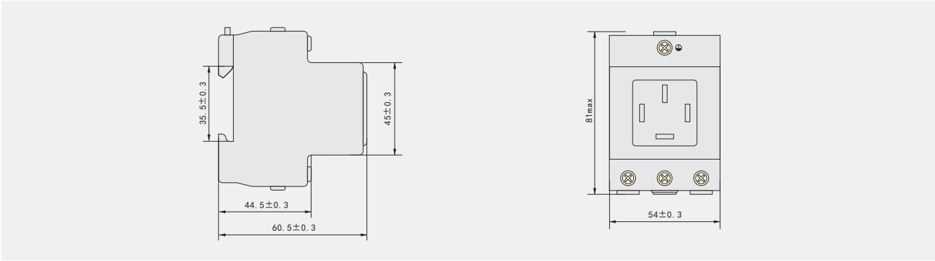
图4、AC30-25/3D 440~外形及安装尺寸
