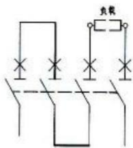
G型接线方式
