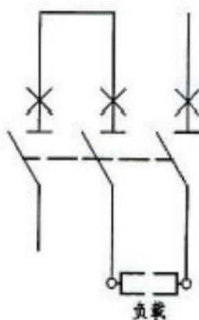
I型接线方式
