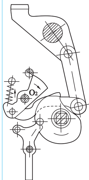
图6 贮能再扣位置
