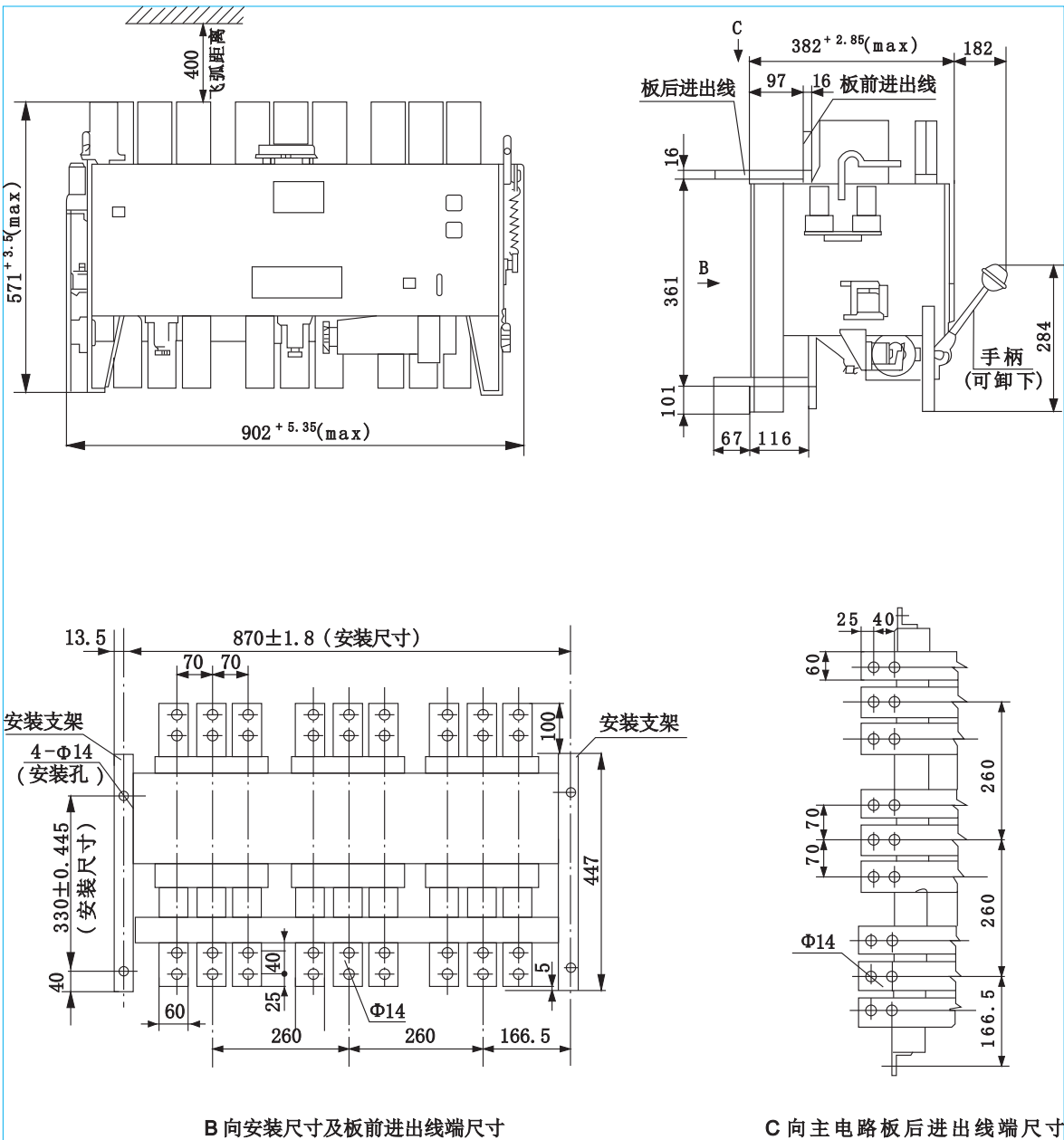
图17 DW15—4000A断路器外形尺寸及安装尺寸图
