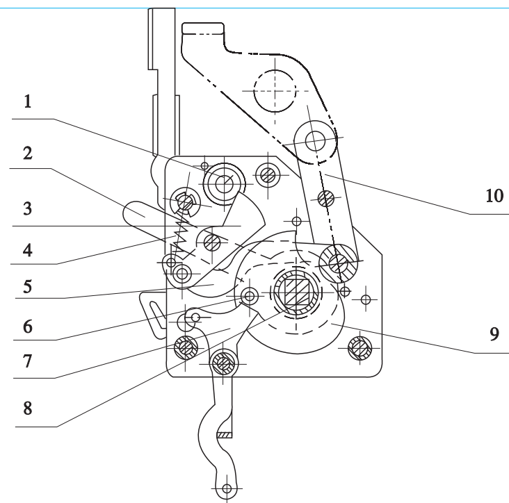
图5 操作机构
