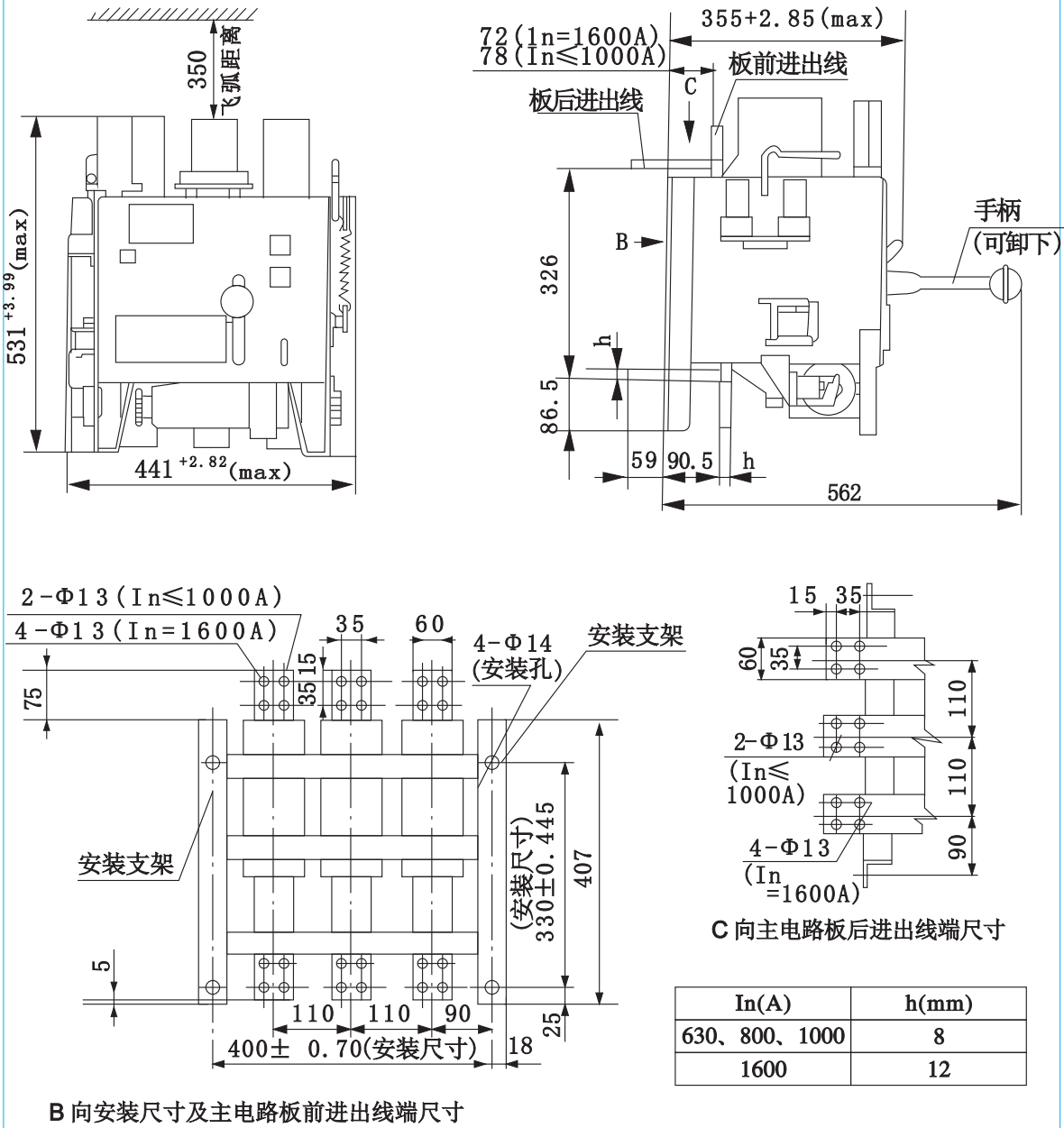
图16 DW15-1600A 断路器外形尺寸及安装尺寸
