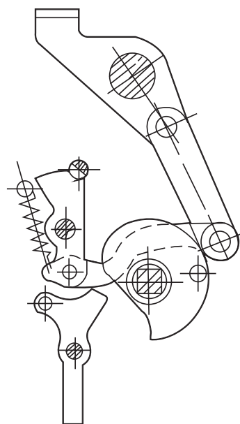
图8 断开位置
