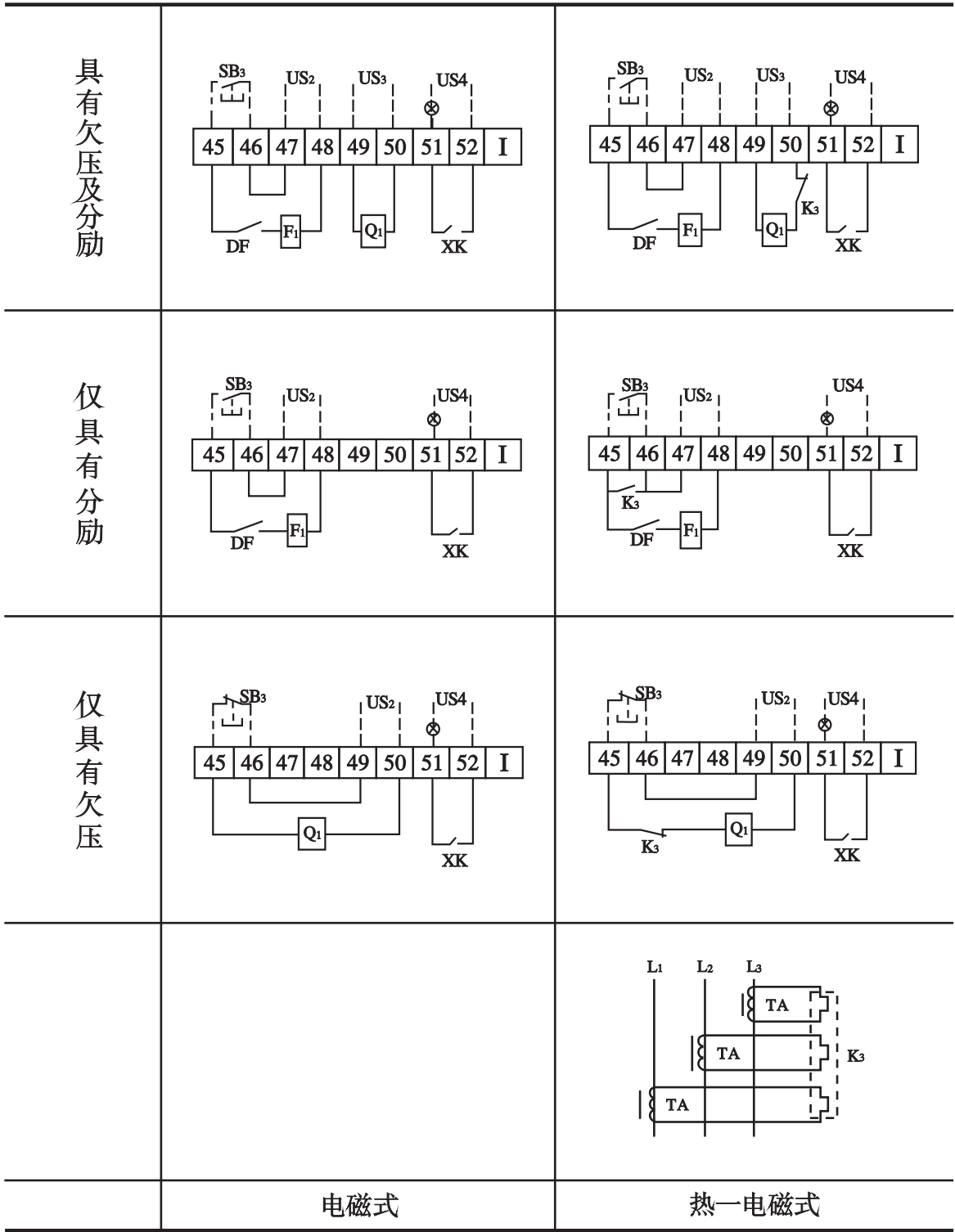
图14 45~52号端子接线图
