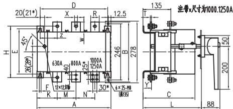
HH15(QSA)-630、800、1000/1250A
