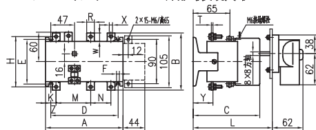
HH15(QSA)-63、125A
