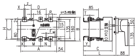
HH15(QSA)-160、250、400A
